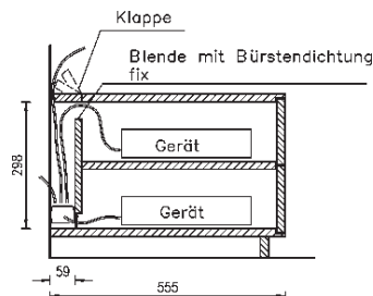
Abb. Kabelmanagement groß
